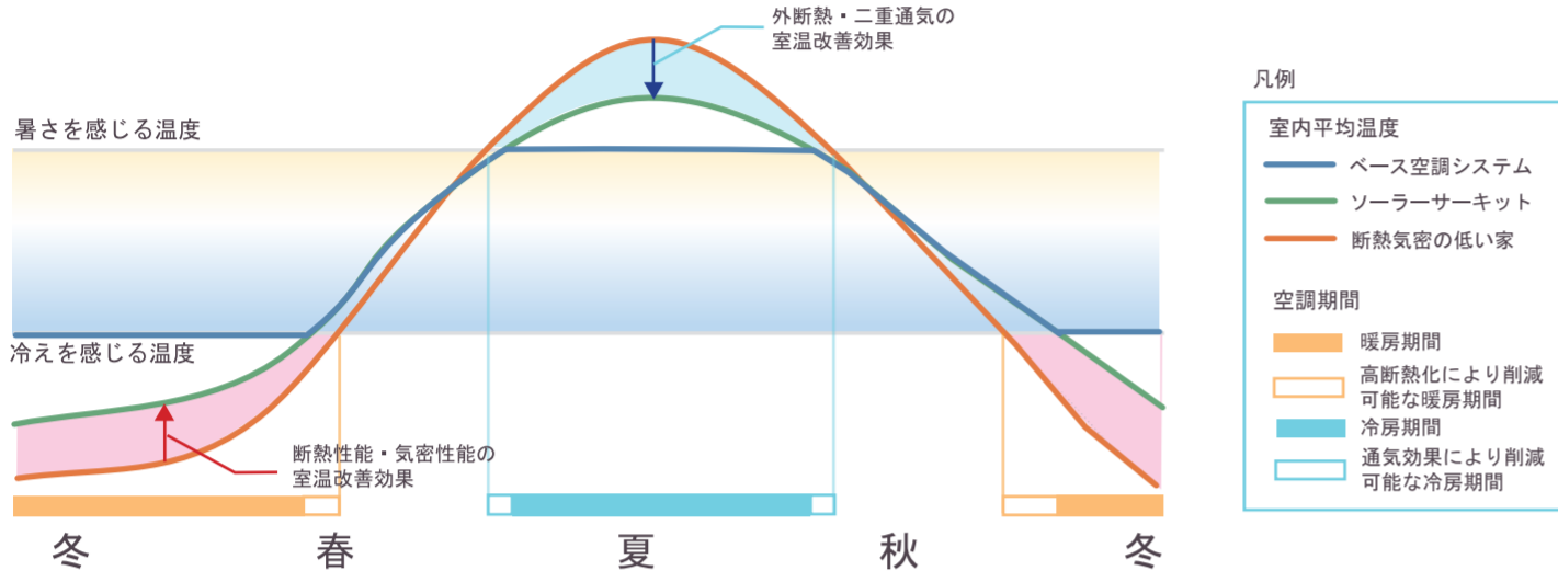
季節の室内平均温度と空調期間イメージ
